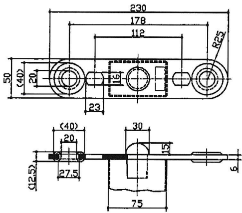
上部詳細図
