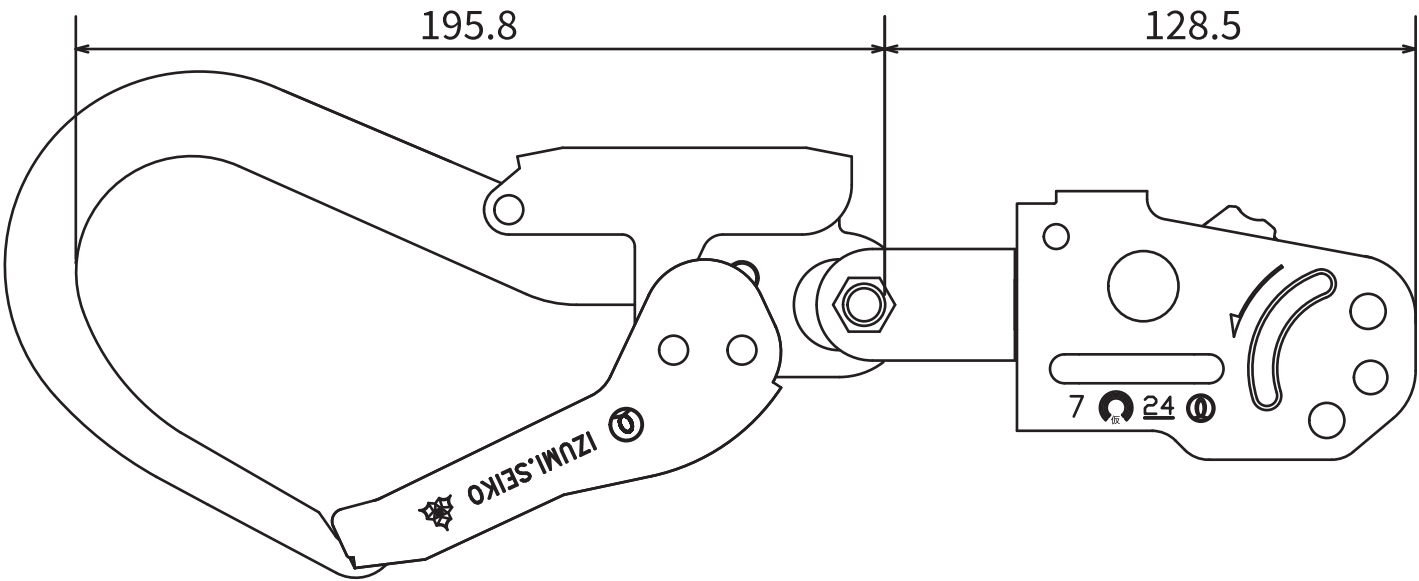
大径フック付緊張器 (ISフック)
